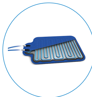
Voda želene temperature teče skozi varjene mikrokanale
